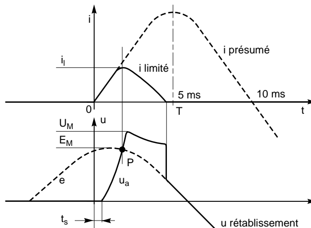
Fig. 4 : courbes u = f(t) et i = f(t) développement de la tension d'arc et sa conséquence : la décroissance du courant de court-circuit.
