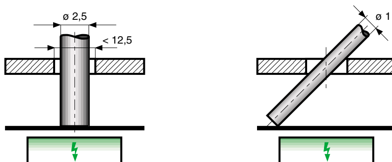
Fig. 2 : un panneau fixe, à l'intérieur de l'enveloppe, empêche le passage des pinces ou « calibres d'essai » de \varnothing 2,5 mm et de \varnothing 1 mm, d'où un degré de protection IP2XD (selon la norme CEI 60529).
